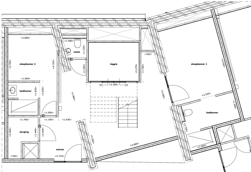
Plattegrond verdieping 03 1:50
